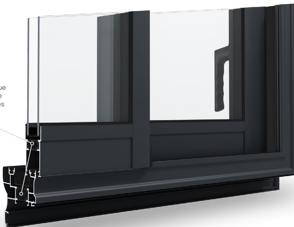
COULISSANT AVEC DORMANT RÉNOVATION Vue extérieure
